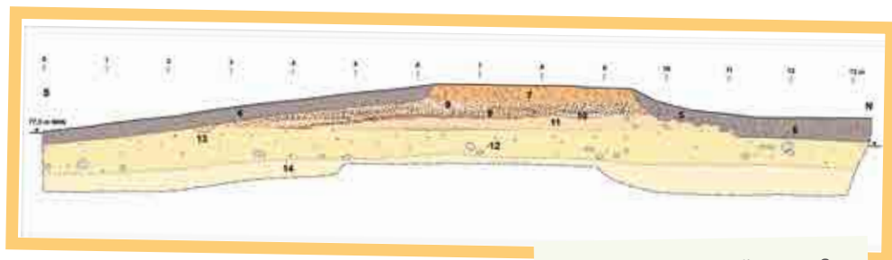
Der Querschnitt der Römerstraße im Klever Reichswald
